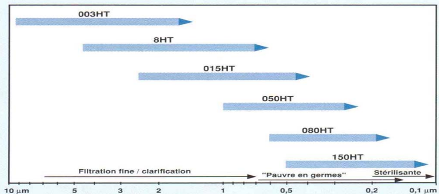
Figure 6 Seuils de rétention Zeta Plus par grade
